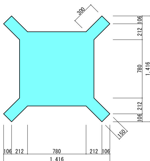
【平面寸法】
