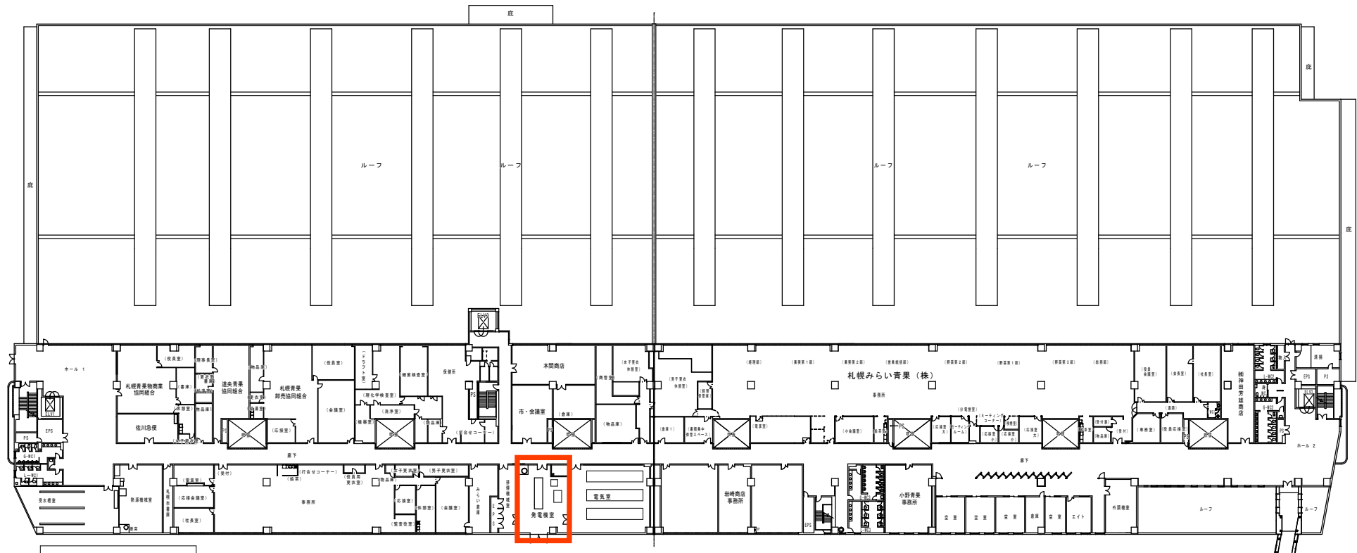
青果棟3階配置図 令和6年12月1日現在
